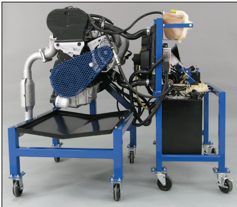
El Entrenador en Reparación de Motores (modelo 90) conectado con el Carro de Arranque del Motor (modelo 91)
